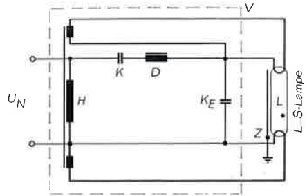
Bild 5. RS-Schaltung kapazitiv
