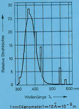
Spektrale Strahlungsverteilung
