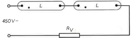
Bild 8. Reihenschaltung für L 20 W/. . G bzw. L 40 W/. . G an Gleichspannung über 450 V
