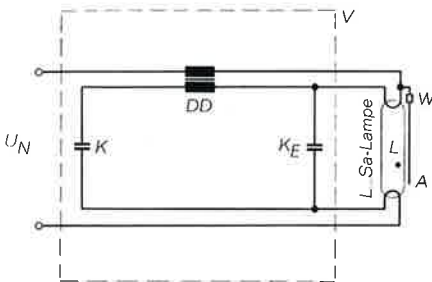
Bild 6. RD-Schaltung
