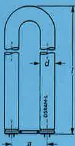
Maß a: 56 mm bei 16 W, 92 mm bei 20 W, 40 W, 65 W
