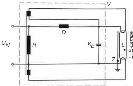
Bild 4. RS-Schaltung induktiv
